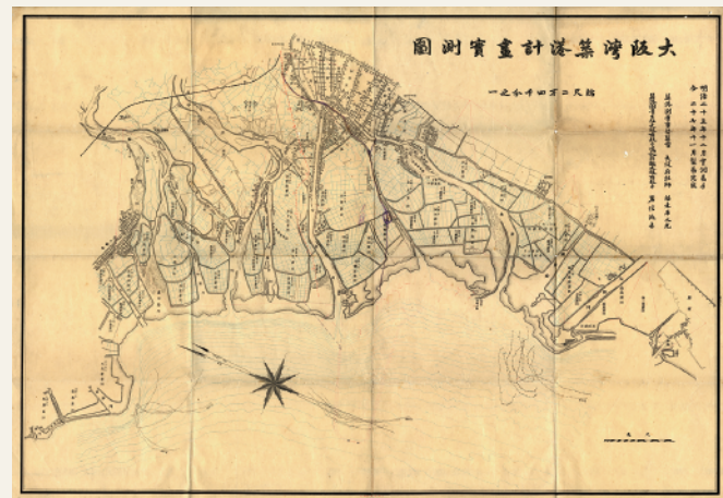
1 大阪湾築港計畫實測圖 15,000円 1枚 明治27年 56×81.4糎 測量事務監督・植木平之允 測量主任・岩佐政吉
